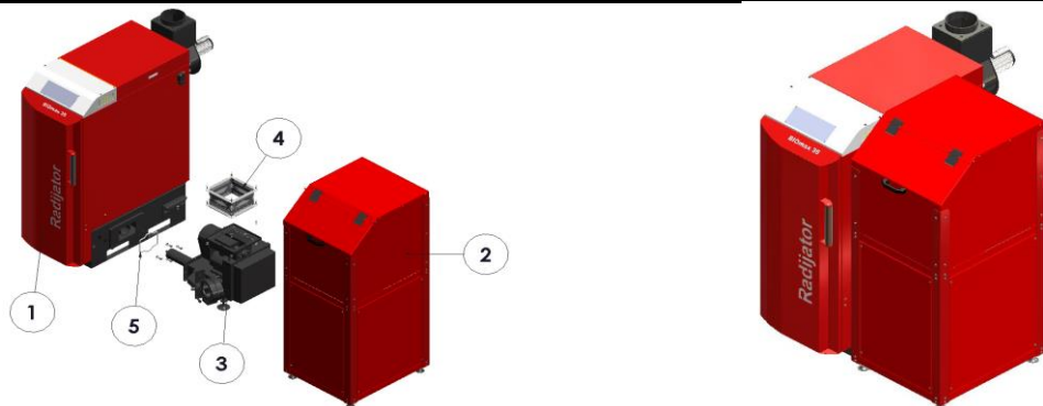
Spisak rezervnih delova za kotao BIOMAX 23.2 & BIOMAX 35.1 / List of spare parts for BIOMAX 23.2 & BIOMAX 35.1
