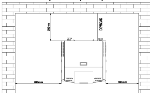
Slika 2: Minimalne udaljenosti kotla od zidova
